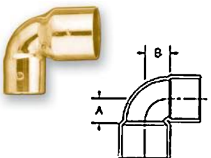
Codos de 90 grados C x C de curva media
