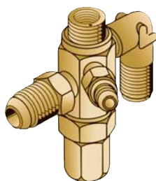
BQE SAE Ecualizadas externamente
